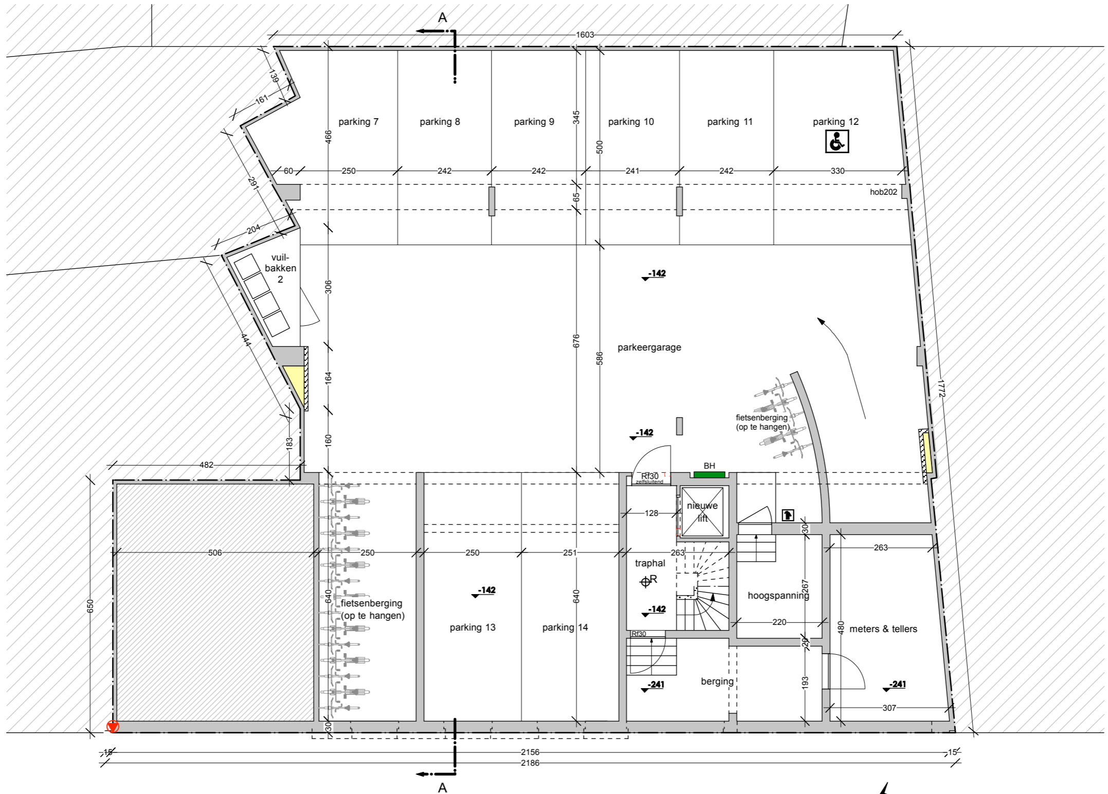
EB 1096: KELDERPLAN nieuwe toestand 1/100
