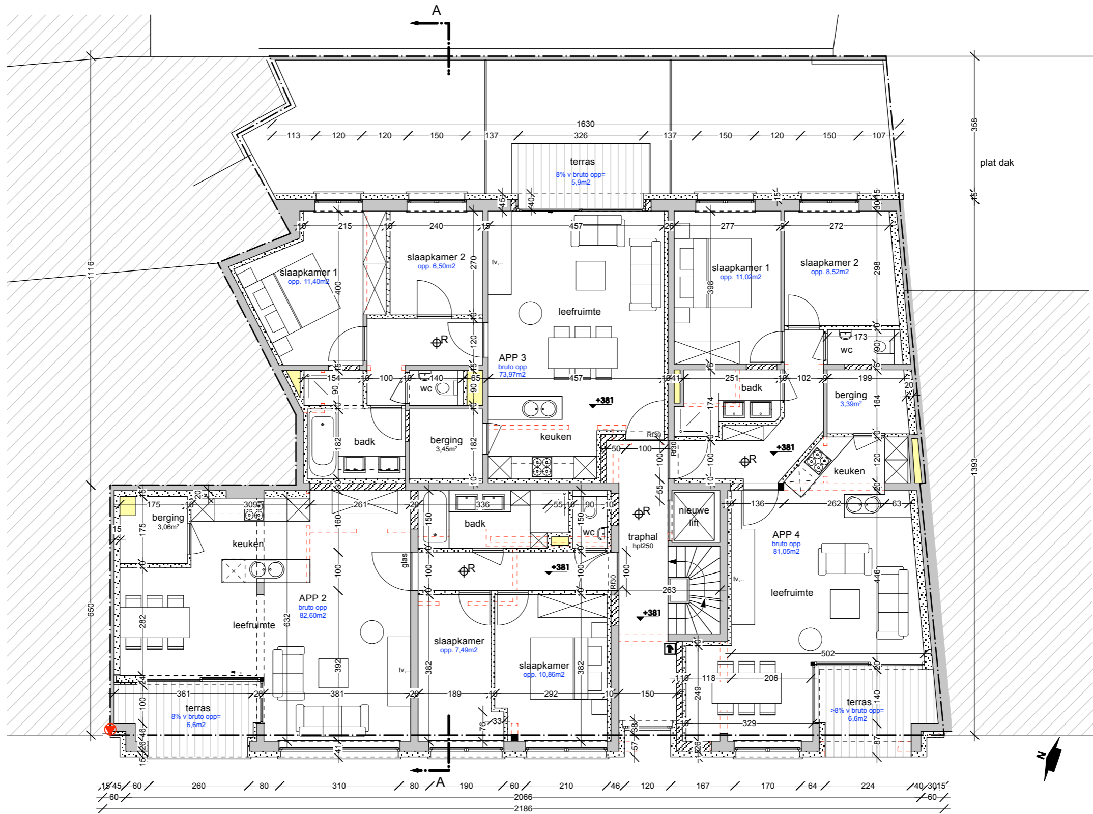
EB 1096: 2e VERDIEPING nieuwe toestand 1/100
