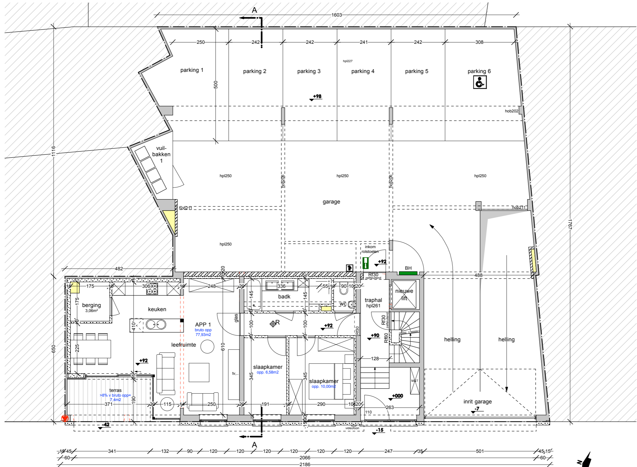
EB 1096: GRONDPLAN nieuwe toestand 1/100
