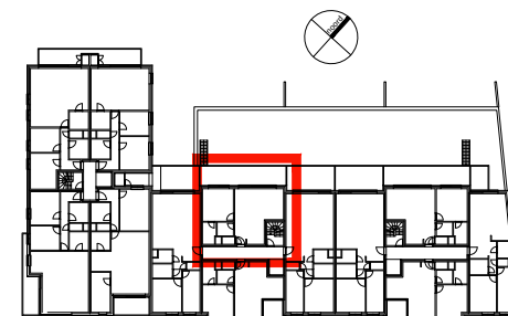
overzichtsplan verdieping 2
