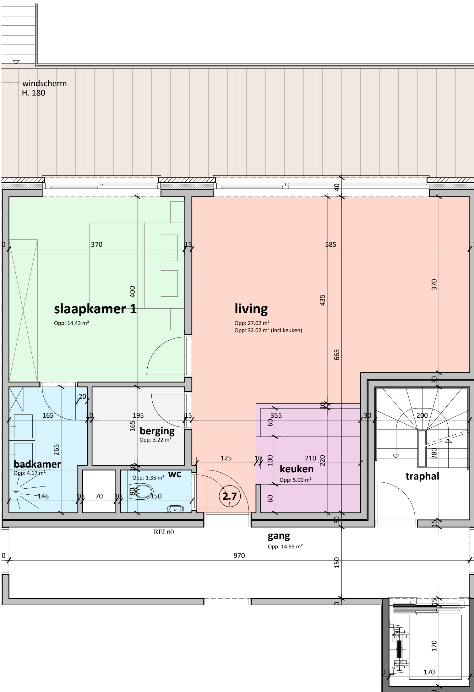
overzichtsplan verdieping 2
