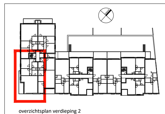
overzichtplan verdieping 2
